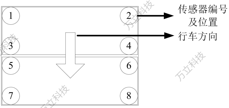
图 6-1 双秤台传感器分布图
