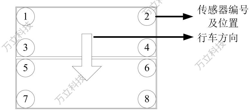
图 6-1 双秤台传感器分布图
