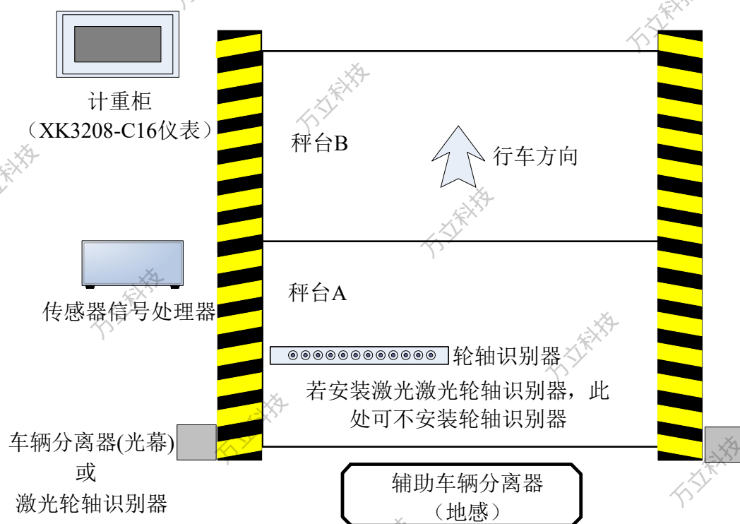
图 3-2 仪表配套产品结构图
