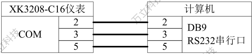
图 4-5 仪表与计算机接线图
