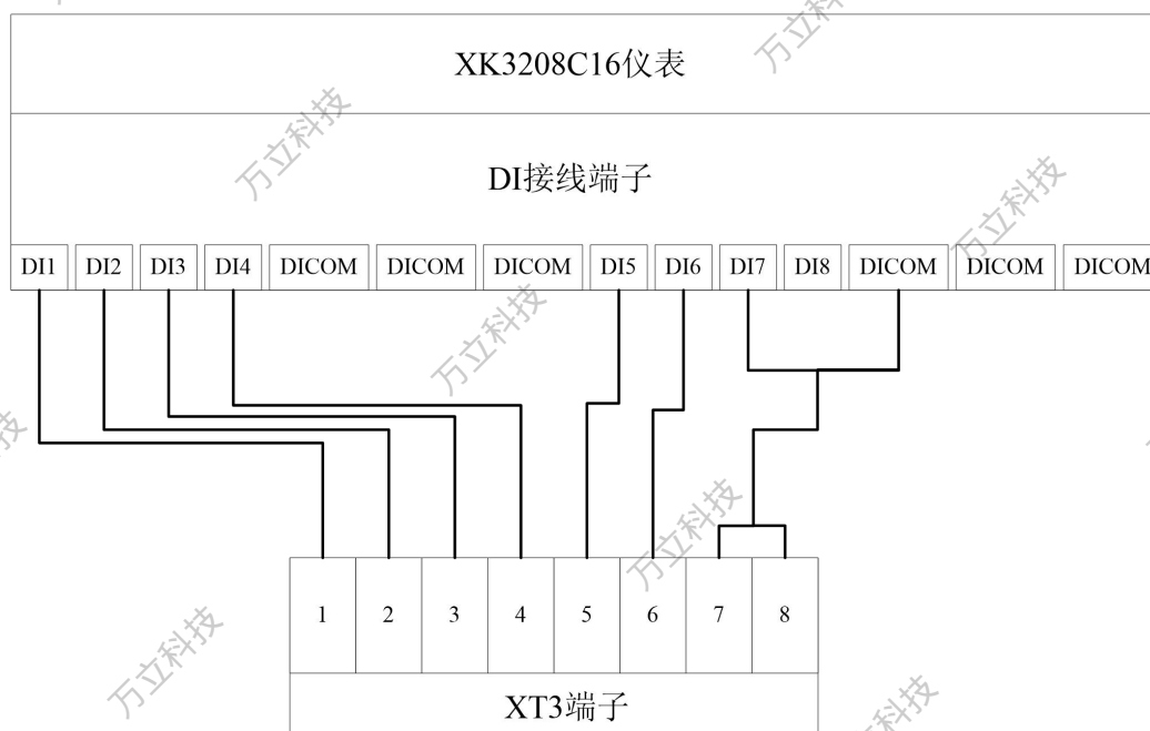
图 6-3 仪表 DI 端子接线图
