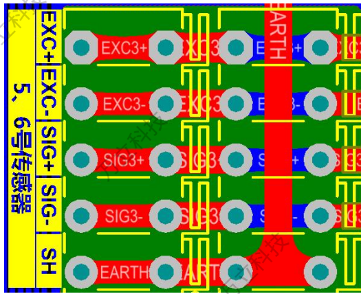
图 6-2 双秤台传感器信号处理器接线图
