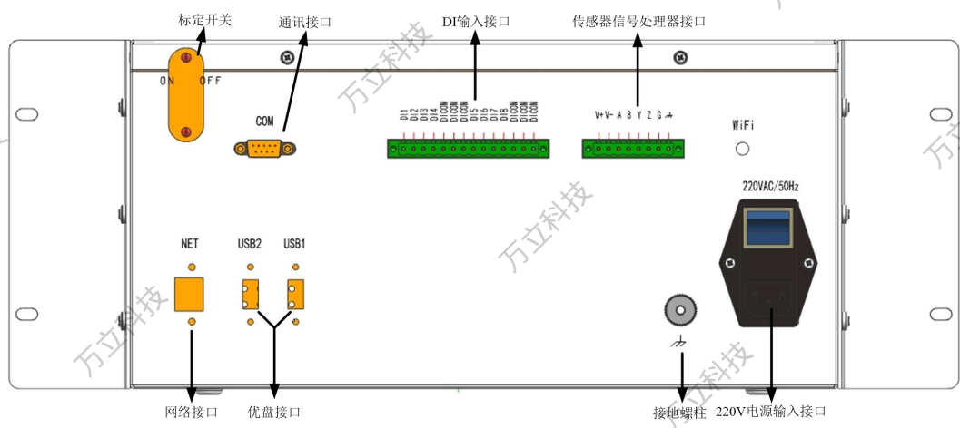
图 4-2 仪表后视图
