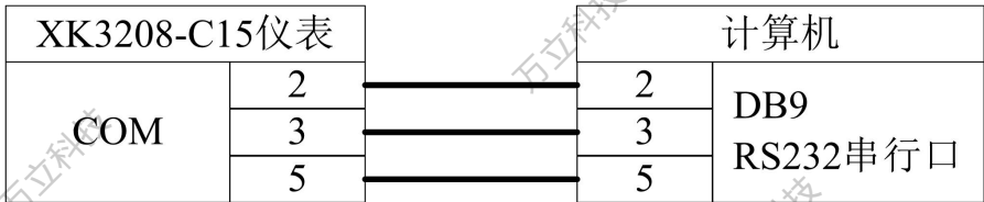
图 4-5 仪表与计算机接线图
