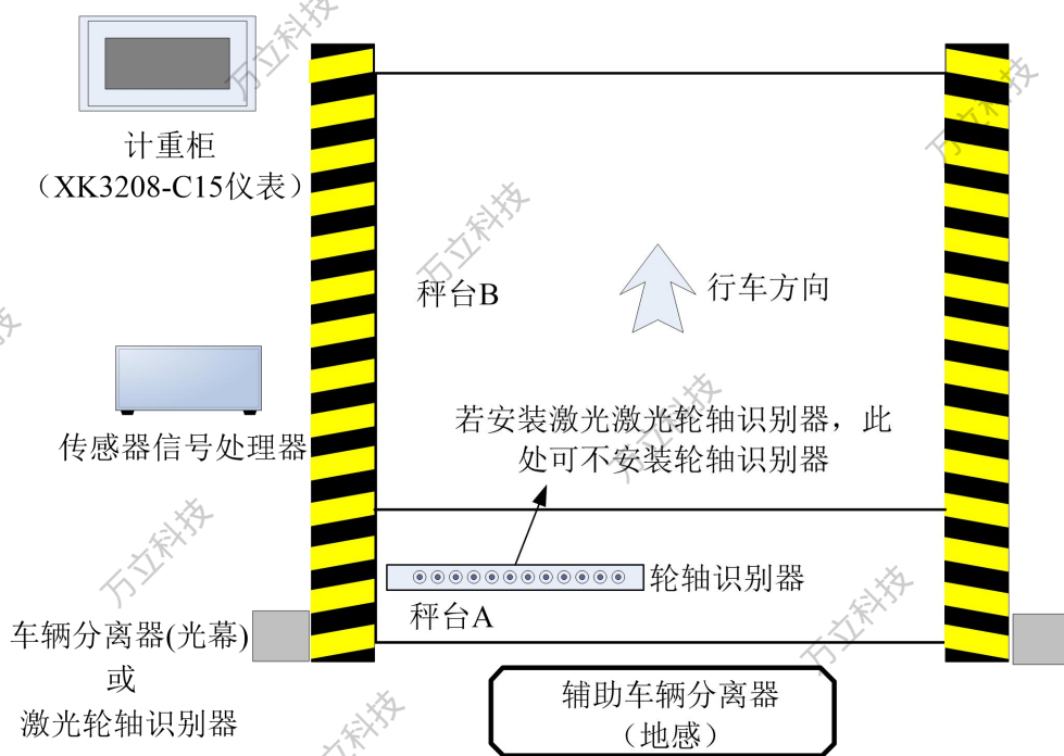
图 3-2 仪表配套产品结构图
