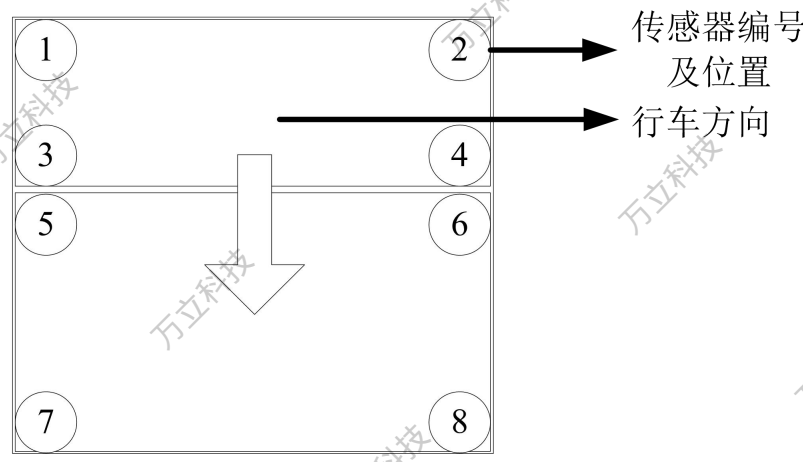
图 6-1 轴组式传感器分布图
