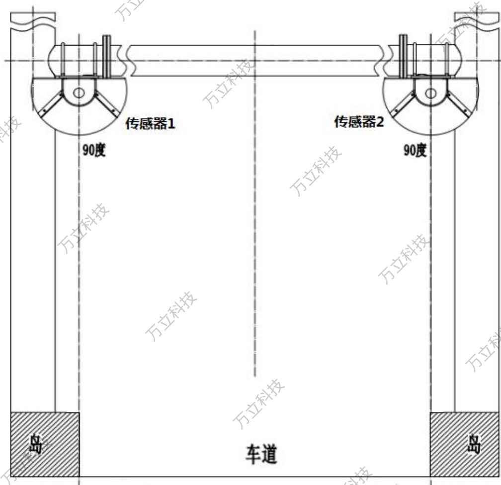
图 5-9 双传感器安装位置主视图
