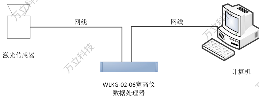
图 3-1 WLKG-02-06 宽高仪数据处理器工作示意图（单传感器）
