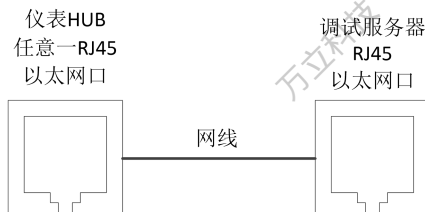
图 4-8 仪表与调试服务器接线图
