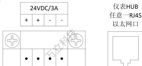
图 4-6 仪表背部传感器供电与通讯接口
