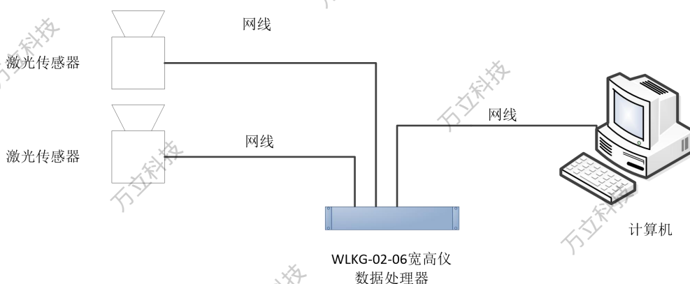
图 3-2 WLKG-02-06 宽高仪数据处理器工作示意图（双传感器）
