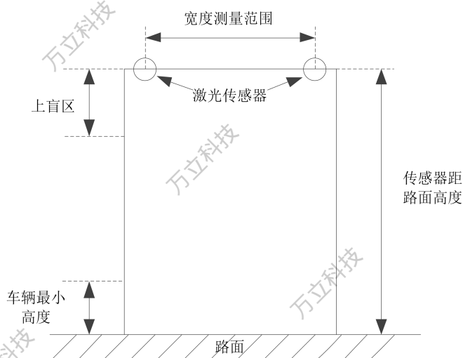
图 5-23 单传感器现场参数示意图
