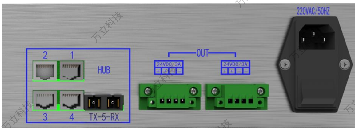
图 4-4 仪表后面板右半部分
