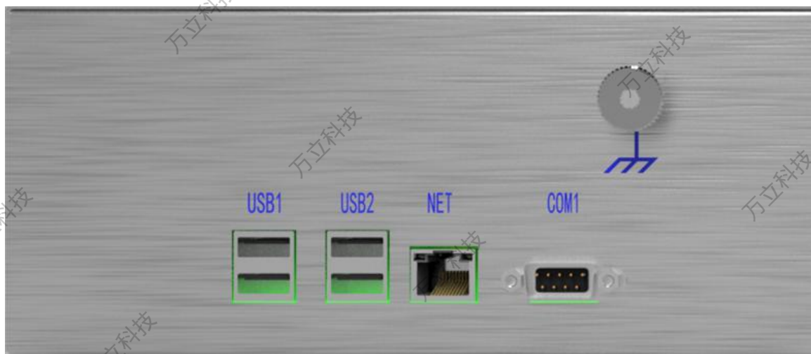
图 4-3 仪表后面板左半部分
