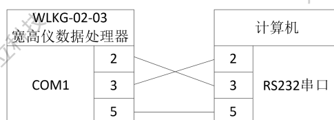
图 7-1 串口通讯连接方式
