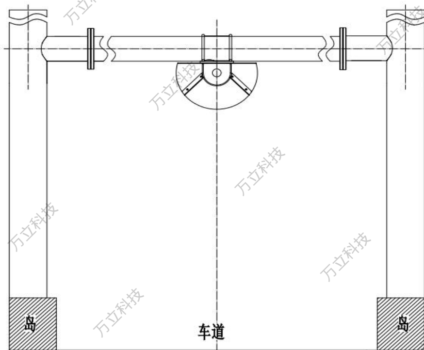
图 5-7 单传感器安装位置主视图
