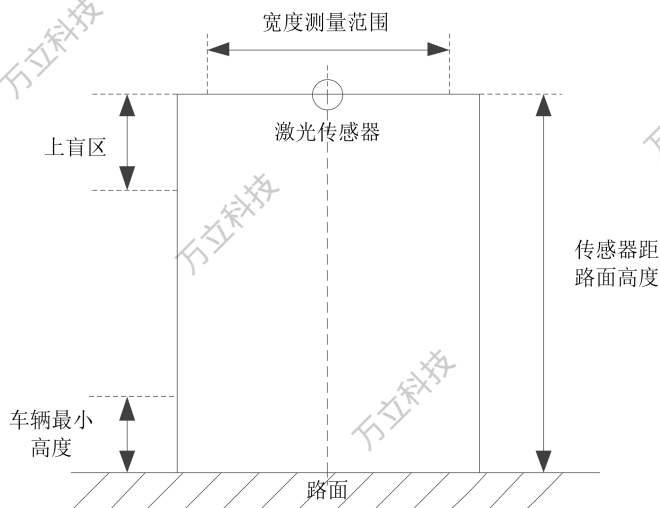
图 5-23 单传感器现场参数示意图
