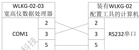
图 4-9 仪表与配置工具计算机连接图
