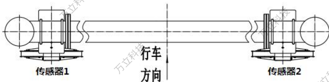
图 5-10 双传感器安装位置俯视图
