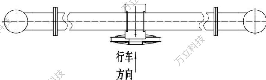
图 5-8 单传感器安装位置俯视图
