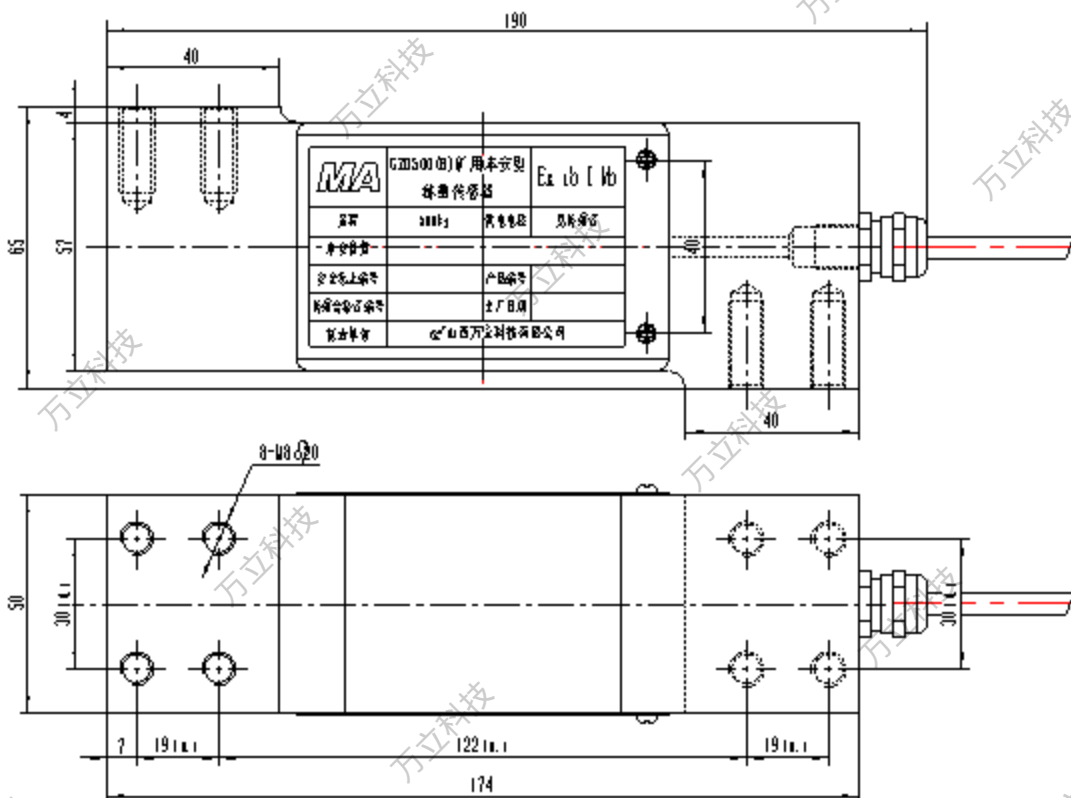
图2 传感器尺寸图
