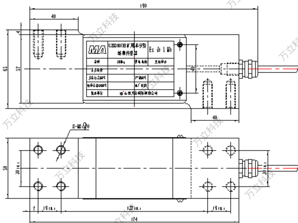
图2 传感器尺寸图
