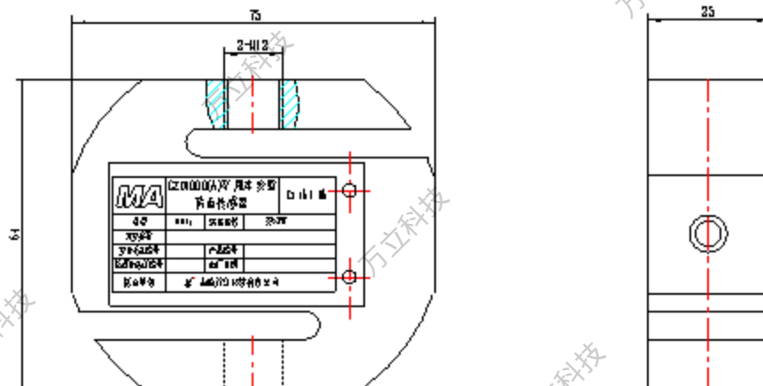
图2 传感器尺寸图
